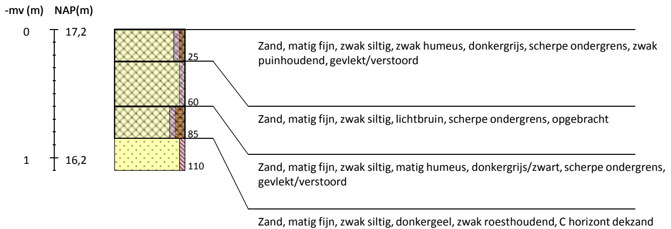
Boring 2 RD-coördinaten: 232781/548895 -
