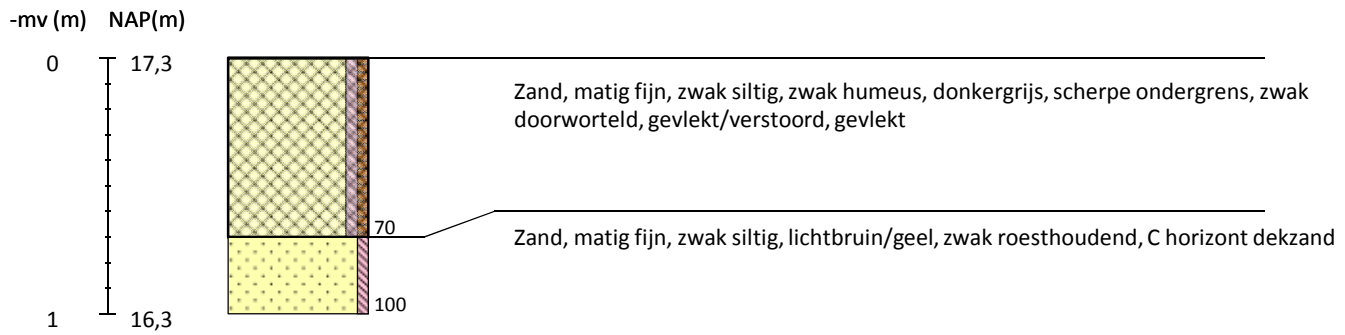
Boring 1 RD-coördinaten: 232798/548894 -
