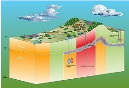
3D zonemodel WKO provincie Drenthe
