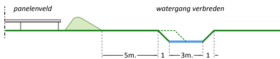
Doorsnede B-B'
