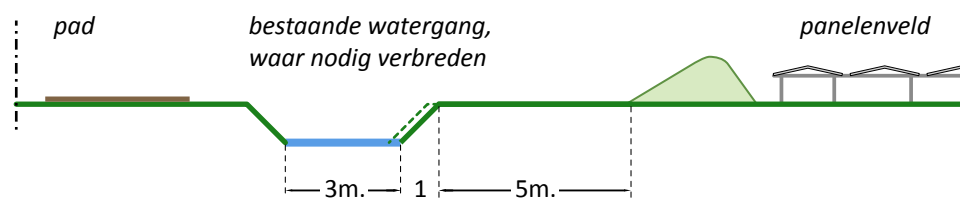
Doorsnede C-C'
