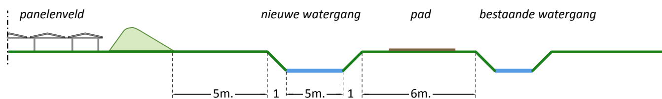
Doorsnede D-D'
