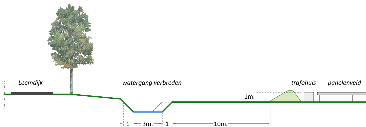
Doorsnede A-A'
